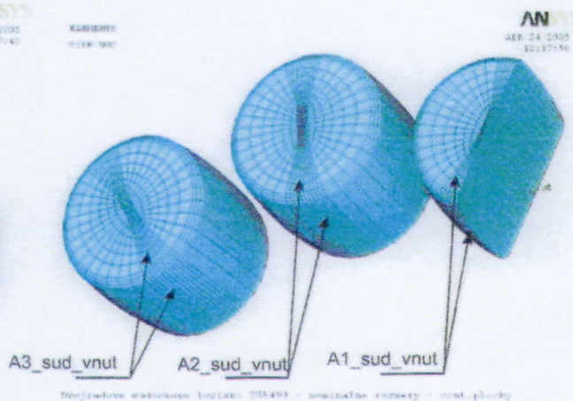
Kontaktné oblasti na valivých telieskach ložiska - oblasti kontakty s vnútorným a vonkajším krúžkom
