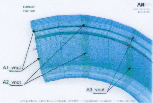
Kontaktné oblasti na vnútornom krúžku
