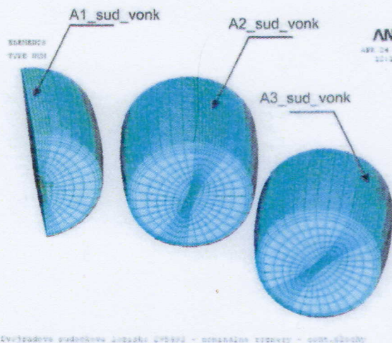
Kontaktné oblasti na valivých telieskach ložiska - oblasti kontakty s vnútorným a vonkajším krúžkom
