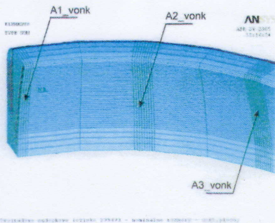
Kontaktné oblasti na vonkajšom krúžku
