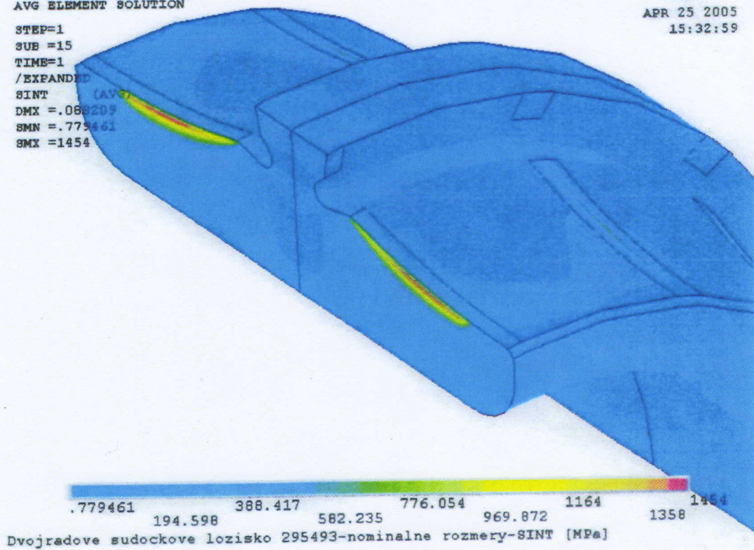
Rozloženie napätí podľa SINT na obežnej dráhe vnútorného krúžku ložiska [MPa]
