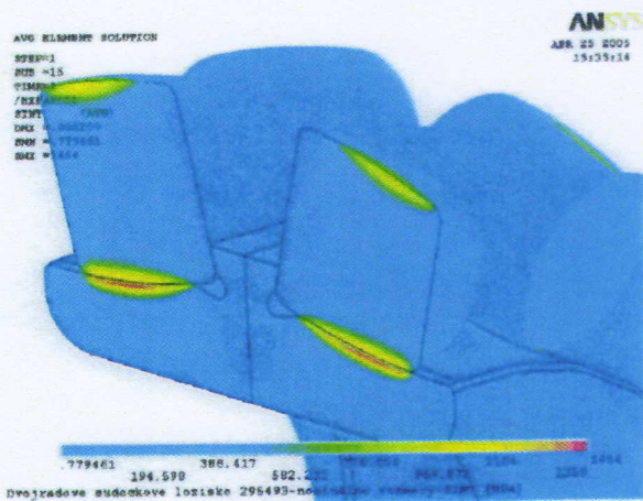
Znázornenie napätí podľa SINT počas kontaktného styku valivých teliesok a vnútorného krúžku ložiska [MPa]
