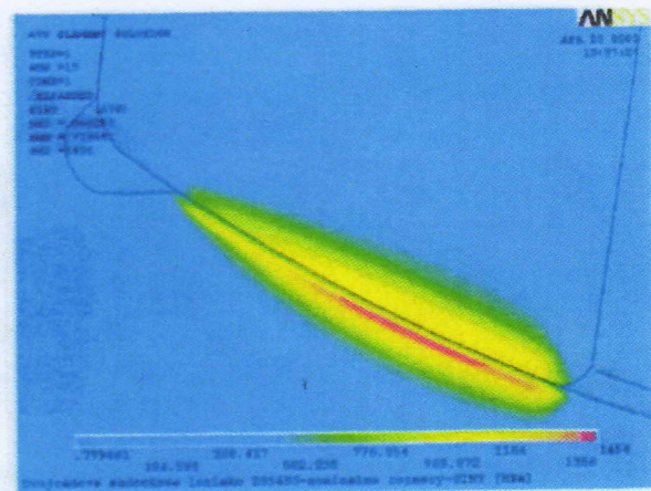
Znázornenie napätí podľa SINT počas kontaktného styku valivých teliesok a vnútorného krúžku ložiska [MPa]
