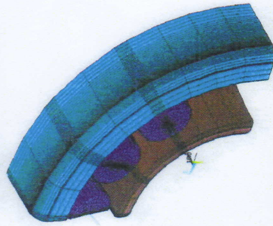
Dvojradowe súdockové ložisko 295493 - nominálne rozmery - FEM model
