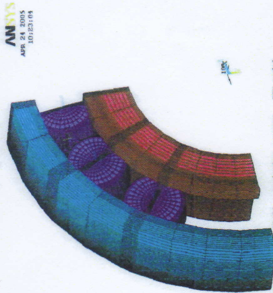
Dvojradowe súdockové ložisko 295493 - nominálne rozmery - FEM model
